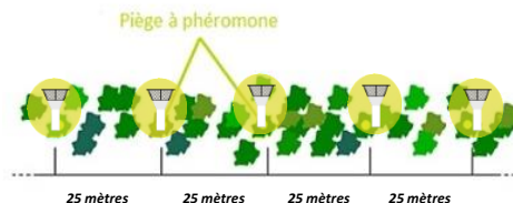
Dispositif de piégeage pour une zone test de 1 hectare
